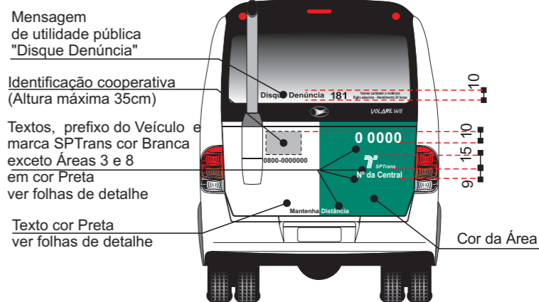
Vista Posterior
