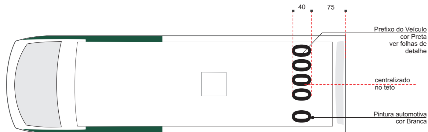
Vista superior
