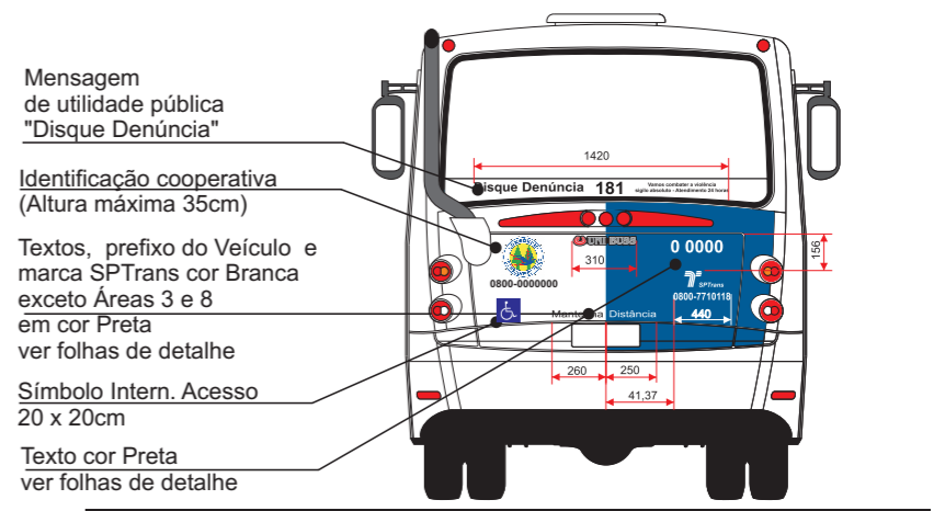
Vista Posterior
