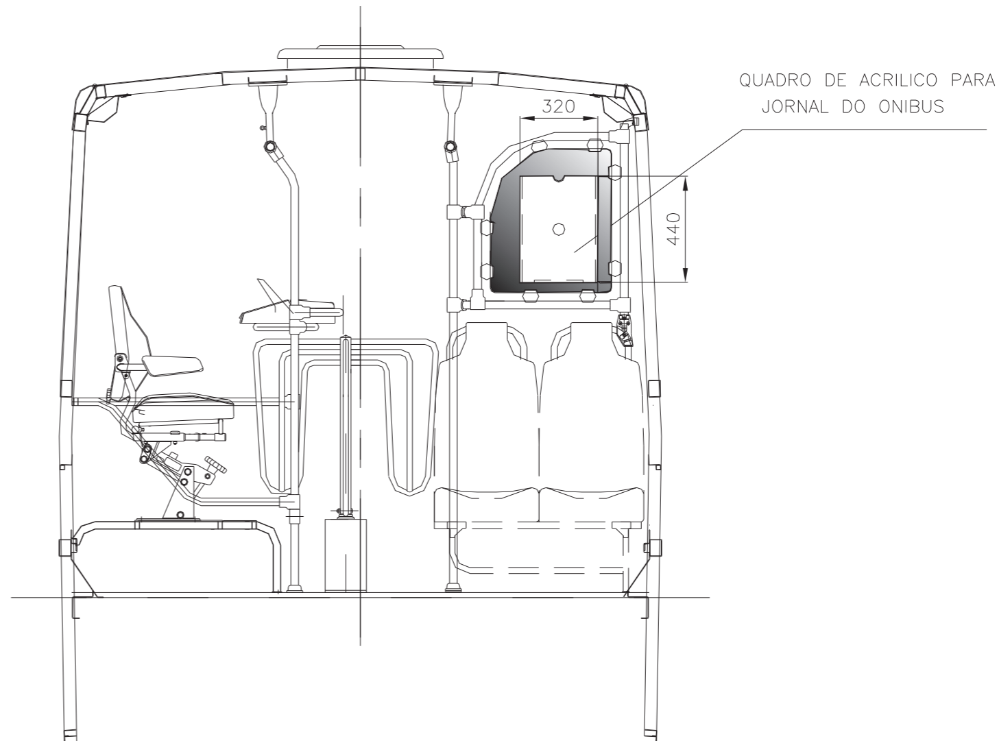
DETALHE DE POSICIONAMENTO DO PORTA CARTAZES NO ANTEPARO (EM FRENTE AO POSTO DE COBRANÇA)
