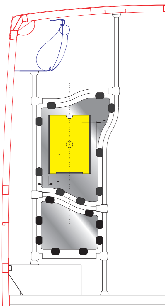
DETALHE DE POSICIONAMENTO DO PORTA CARTAZES NO ANTEPARO (ATRÁS DO MOTORISTA)
